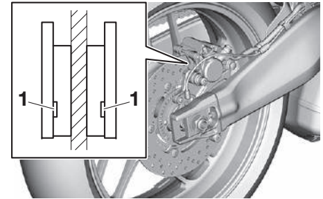
1. 煞車片磨耗指示溝槽
