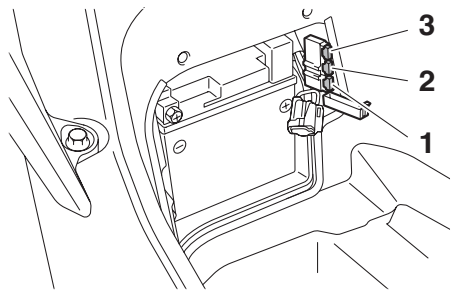
1. MAIN 主保險絲 2. USB_ASSY 保險絲 3. 備用保險絲
