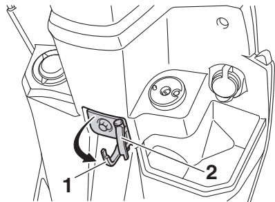
1. 前置物掛鉤 2. 扣環
