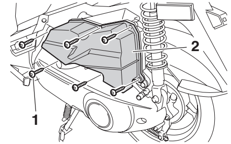
1. 螺絲(x6) 2. 空氣濾清器蓋
