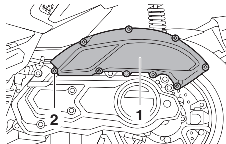
1. 空氣濾清器箱蓋 2. 螺絲(x9)
